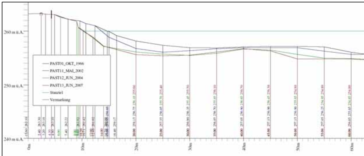
Abbildung 6: Zeitliche Entwicklung der Enns-Sohle im Unterwasser KW Mühlrading bei Fluss-km 13,450. Schwarz: 1966; Blau: 2002; Grün: 2004; Rot: 2007; Quelle: Ennskraft.
