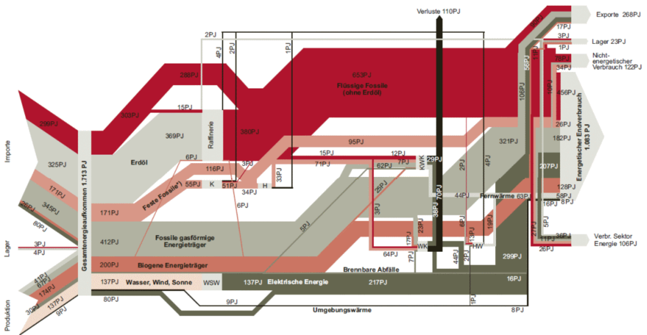
Energieflussbild Österreich 2007
