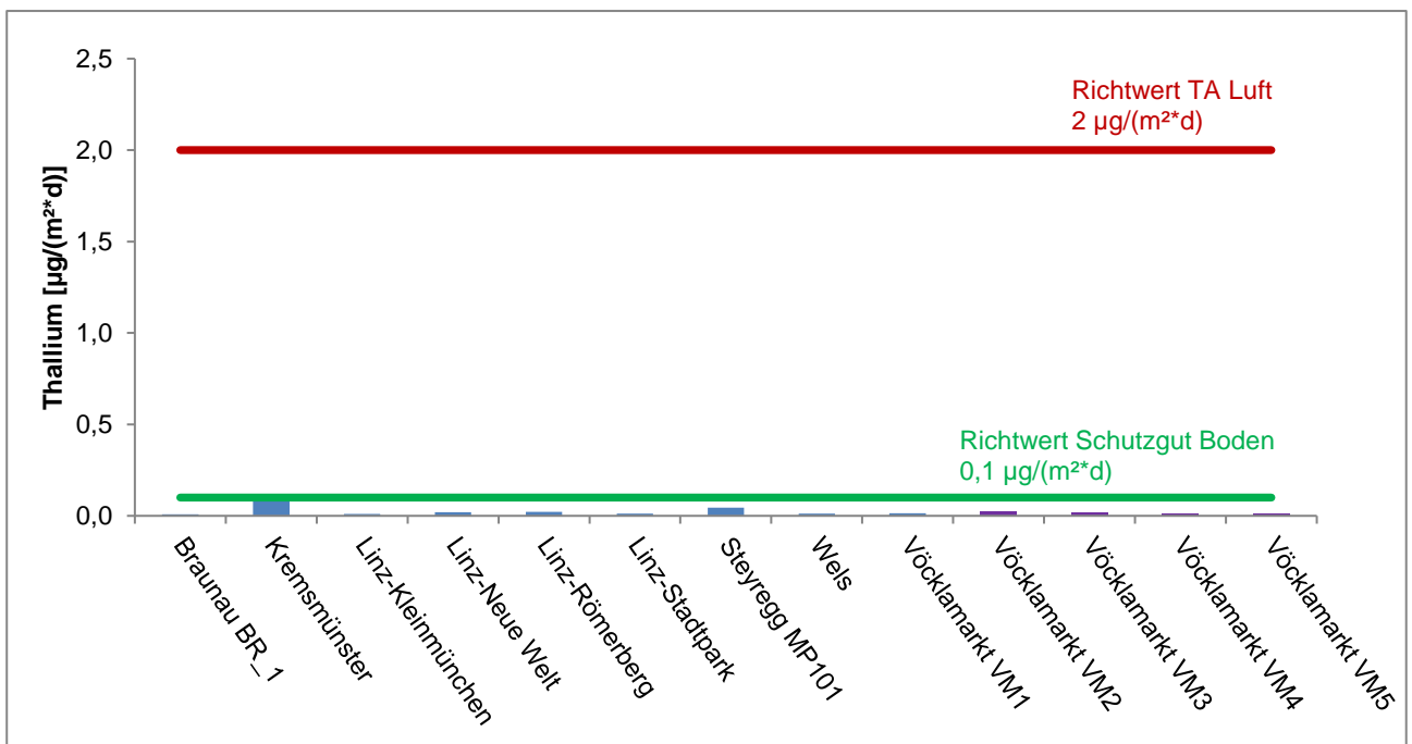
Abbildung 13: Thallium im JMW im Vergleich zu den Oö. Messstellen 2024
