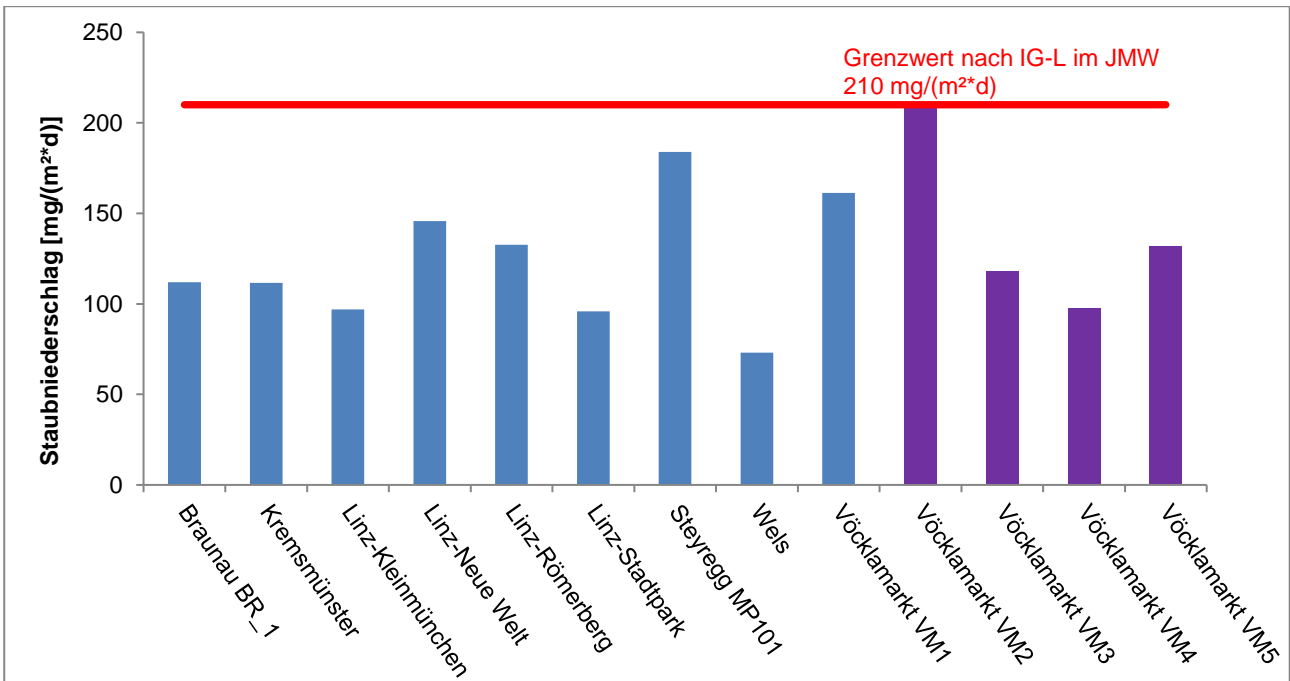
Abbildung 7: Staubniederschlag im JMW in Vöcklamarkt im Vergleich zu den Oö. Messstellen 2024
