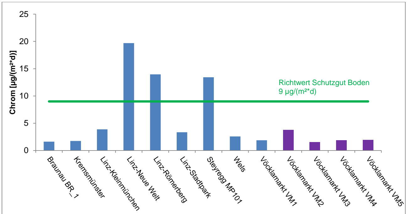
Abbildung 12: Chrom im JMW im Vergleich zu den Oö. Messstellen 2024
