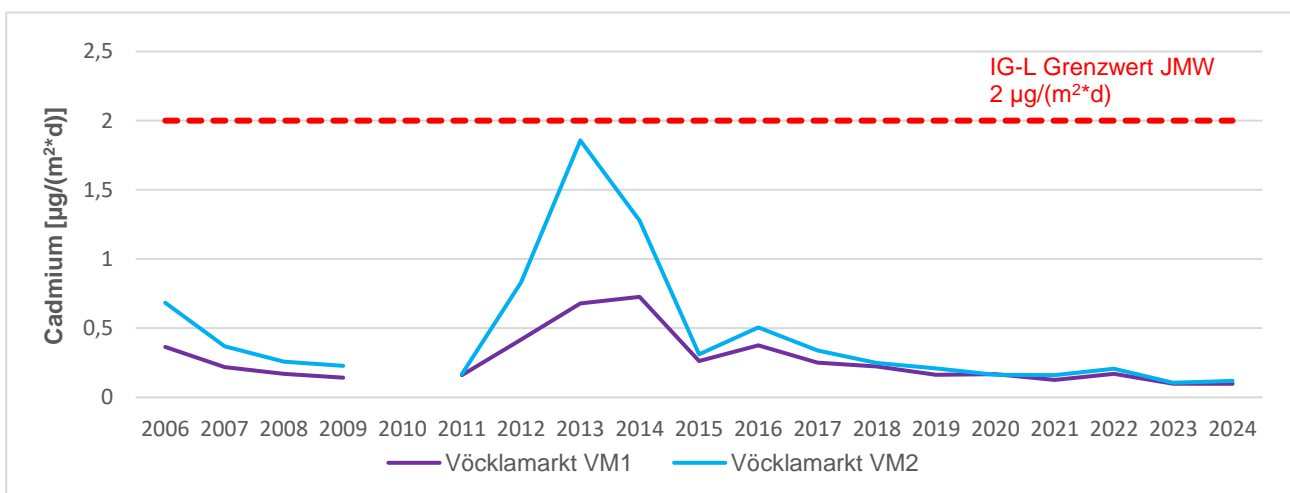
Abbildung 20: Cadmium im JMW im Jahrestrend 2006 – 2009 und 2011 – 2024
